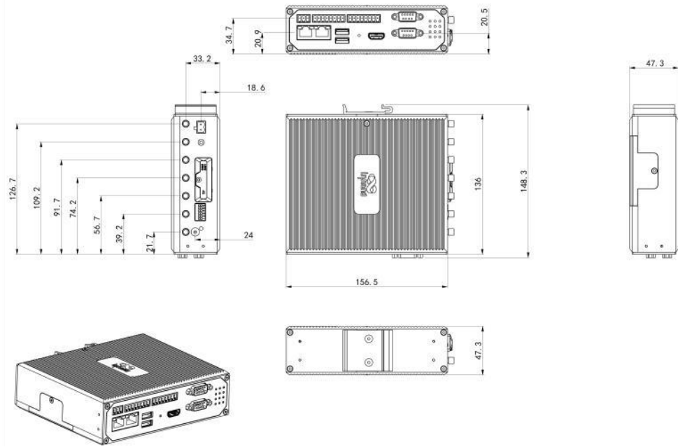
EC942 导轨方式
