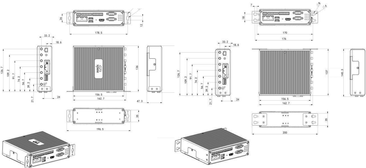
EC942 壁挂方式A*
